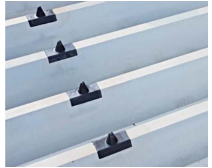
キャップマン取付け状況
