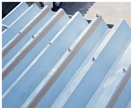
カシメ部両面テープ(5640)張り付け状況
