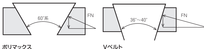
図5 側壁垂直力の比較
