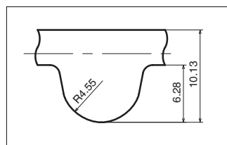
GH14M Standardriemenbreite
