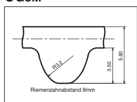
G8M Standardriemenbreite
