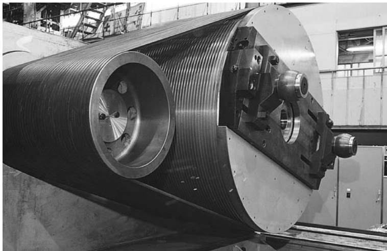
Hochleistungspoliergerät (MAXSTAR WEDGE Keilriemen)
