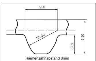
Standardriemenbreite
