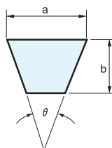
PRENE Keilseil
