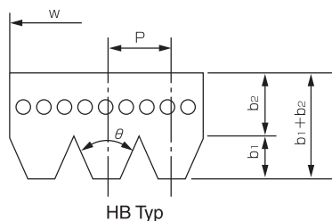
HB Typ
