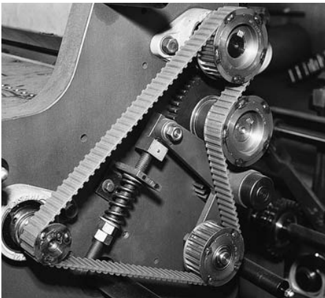
Verpackungsmaschinen (Polyurethananer Doppelzahnriemen)
