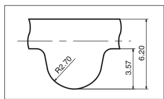
H8M Standardriemenbreite
