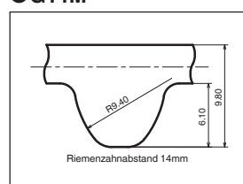
G14M Standardriemenbreite
