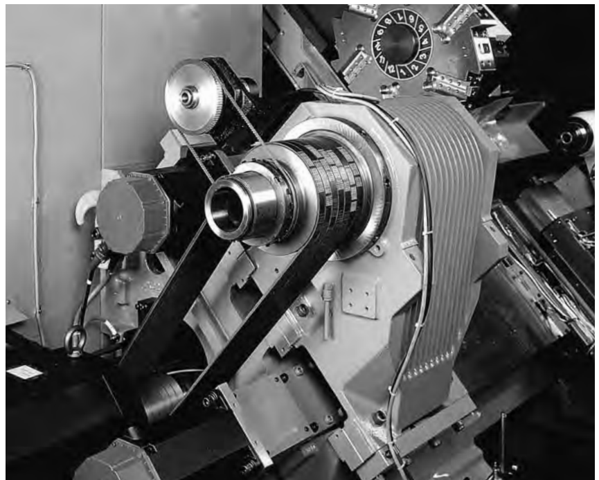
NC旋盤(リブスター®ベルトG)
