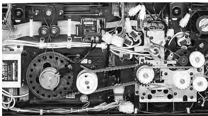
複写機(タイミングベルトG)
