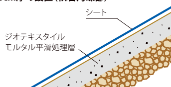
ニ) モルタル平滑処理層 5~10cm厚の設置 (軟岩角礫部)
