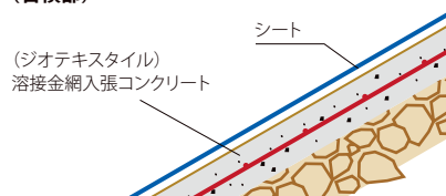
ホ) 溶接金網入10cm厚の設置 (石積部)
