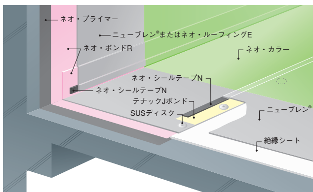
[NB-401MJ 平場全面機械的固定工法]
