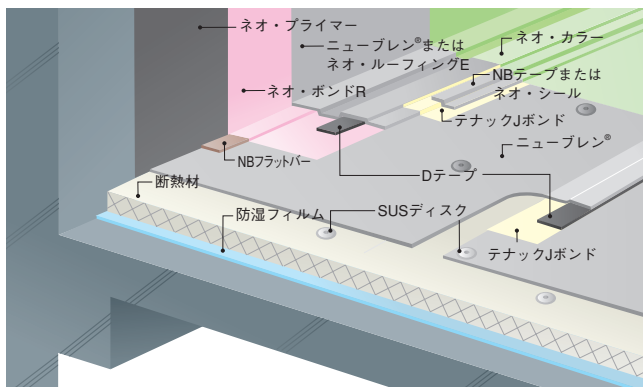
[NB-401MJ 平場全面機械的固定工法]
