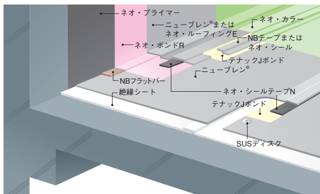
[NB-101MJ 平場全面機械的固定工法]
