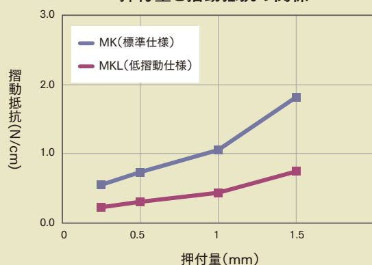
押付量と摺動抵抗の関係
